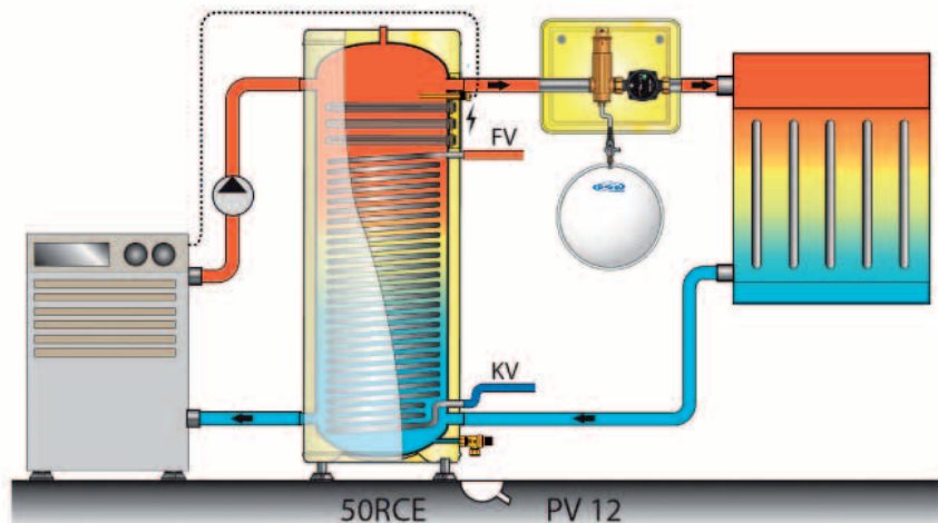
PUSKURIVARAAJAA 50RCE, KIERUKALLINEN JA VASTUKSELLINEN VARAAJA, LÄMPÖPUMPPUUN KYTKETTYNÄ
