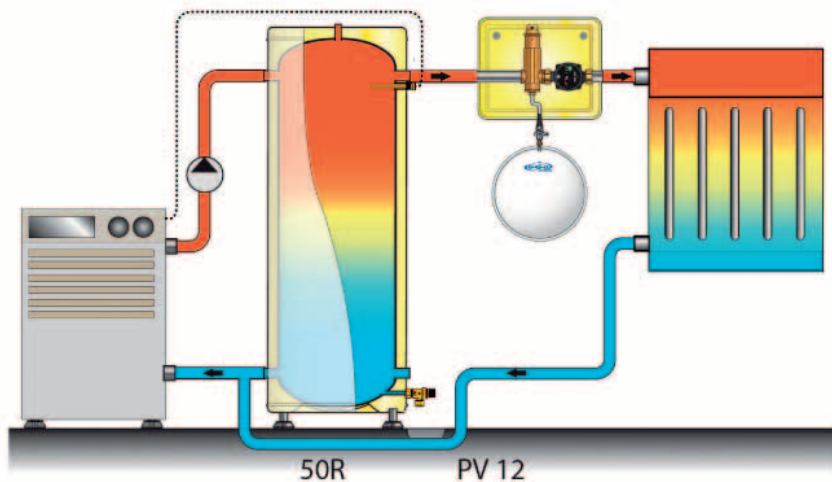
PUSKURIVARAAJA 50R LÄMPÖPUMPPUUN KYTKETTYNÄ
